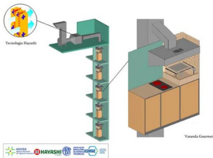
Sistema de Exaustão Varanda Gourmet
