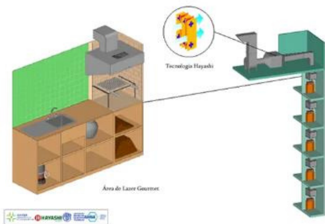
Sistema de Exaustão Área de Lazer Gourmet
